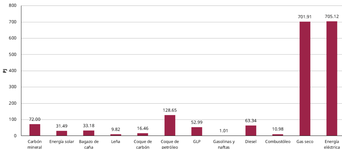
Figura 5.6 Composición del consumo de energía del sector industrial por energético, 2024
