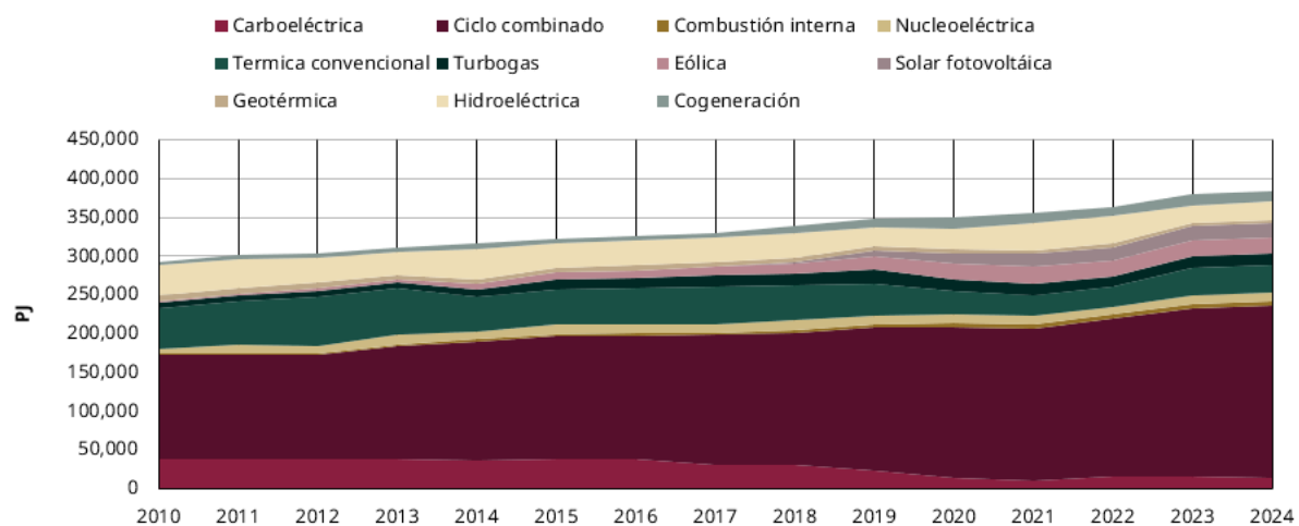
Figura 4.6 Evolución de la generación bruta de energía eléctrica por tecnología, 2010-2024
