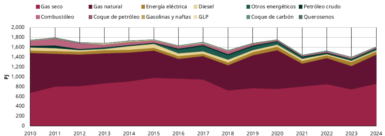
Figura 4.7 Evolución del consumo propio del sector por energético, 2010 - 2024
