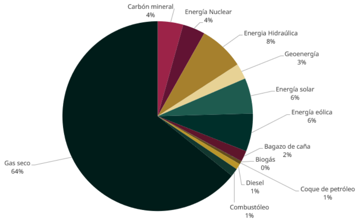
Figura 4.5 Energéticos empleados para la generación de energía eléctrica, 2024
