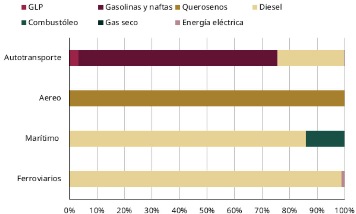
Figura 5.18 Estructura del consumo de energía de subsectores en el sector transporte, 2010-2024
